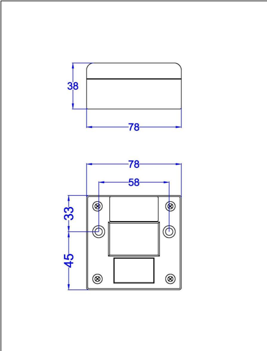
Figure 1. Encombrements généraux
