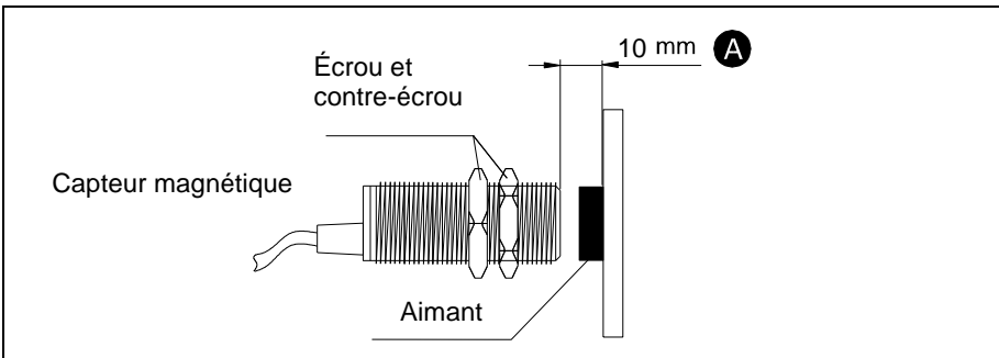
Figure 3. Position typique du capteur magnétique D.12 code 671.
